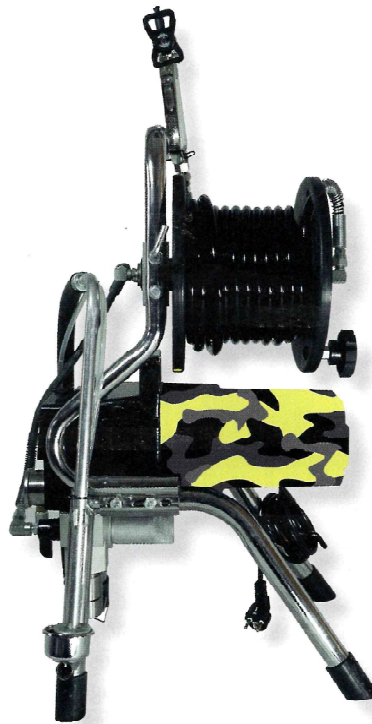
8 Das Monster EasySpray 2.2 ist eine verschleißarme EasySpray-Materialpumpe ohne Zylinder mit feststehenden und nachjustierenden Dichtpackungen für lange Standzeiten und geringe Wartungskosten. Foto: Linz
